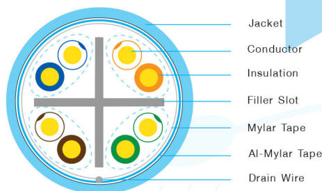
US-9266LSZH
